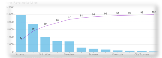
Pareto
